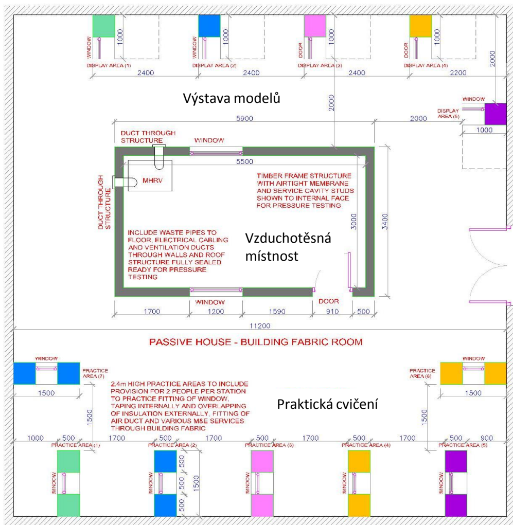
Půdorys školícího centra
