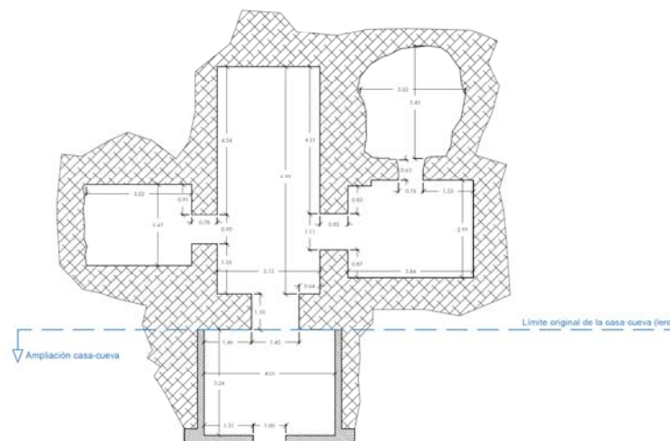
PLANTA CASA CUEVA UNA VEZ REALIZADAS LAS EXCAVACIONES Y AMPLIACIÓN PLANTEADA
